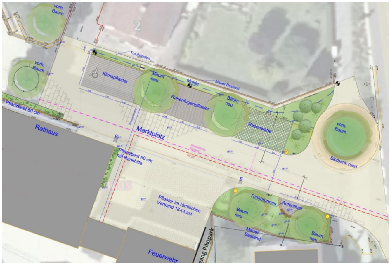
Entwurf Klimamusterparkplatz
